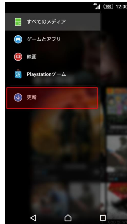
Android5.0（更新後）
