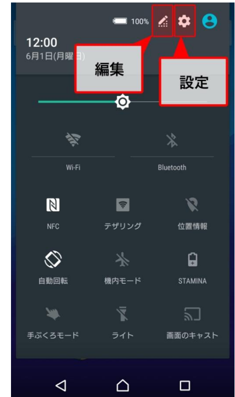
Android5.0（更新後）
