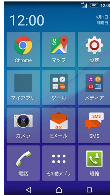
Android5.0（更新後）
