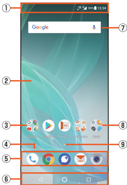
《Home screen》
