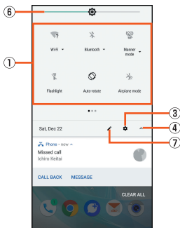
《Status panel》
