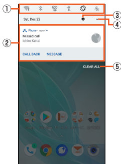
《Notification panel》
