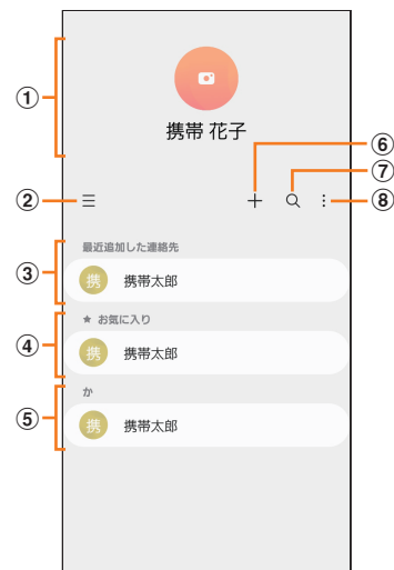
《連絡先画面》
